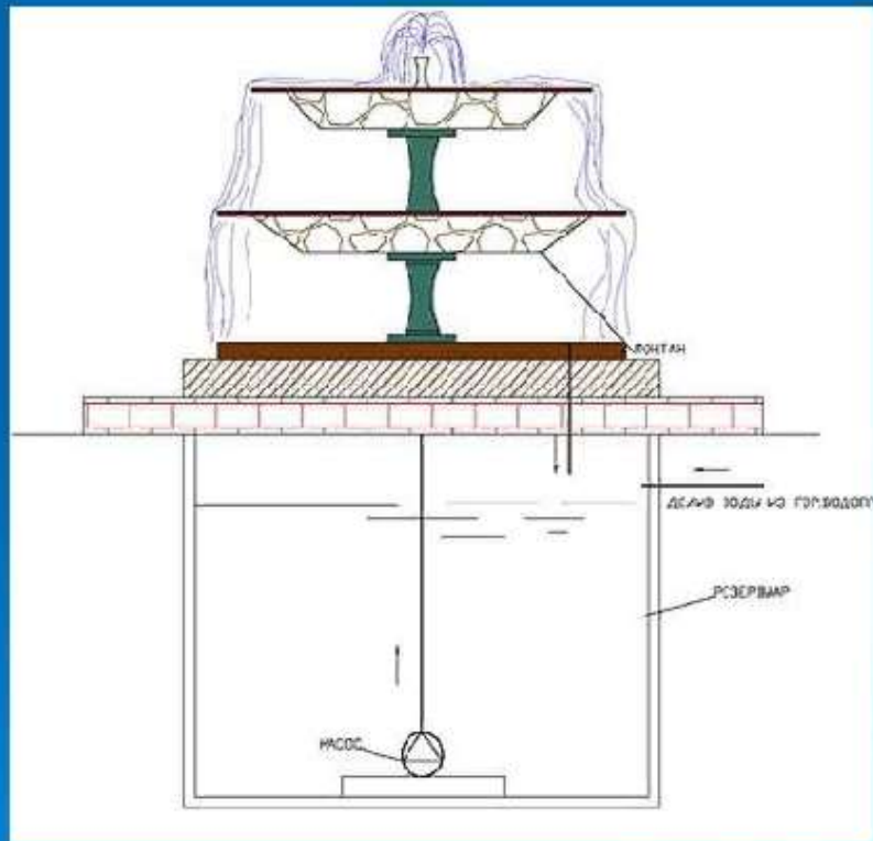
ПОПЕРЕЧНЫЙ РАЗРЕЗ ФОНТАНА В ВИДЕ ЛЕСТНИЦЫ
