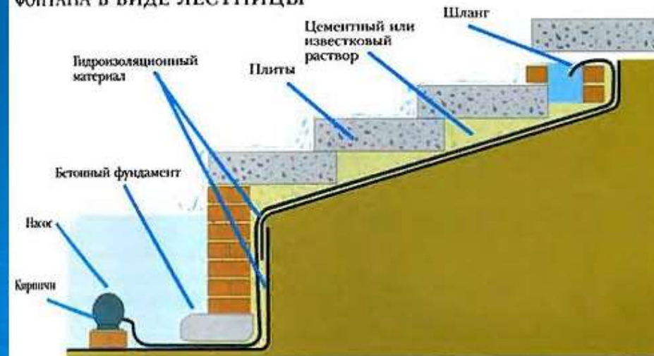
ПОПЕРЕЧНЫЙ РАЗРЕЗ ФОНТАНА В ВИДЕ ЛЕСТНИЦЫ
